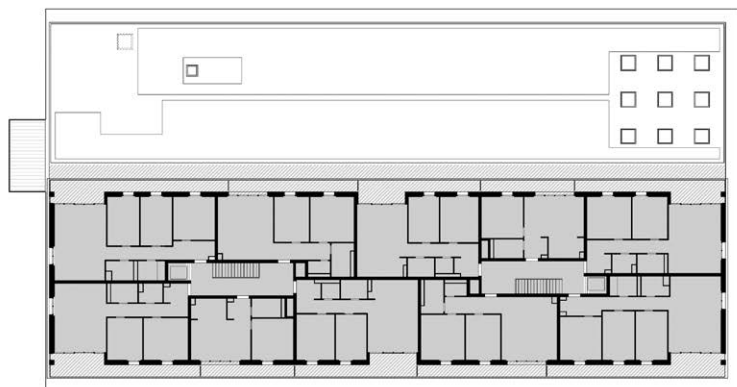
Bâtiment D, plan niveau 01
