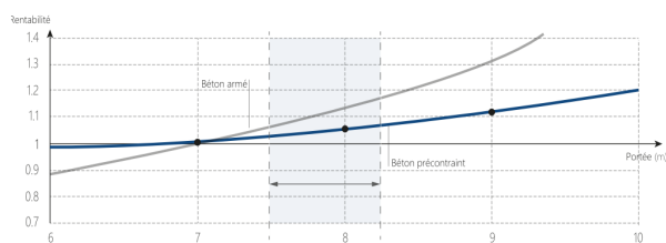
Comparatif du coût de construction de dalle en fonction de la portée
